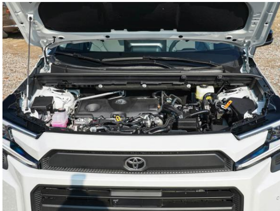
Compartimiento del motor (frontal)
